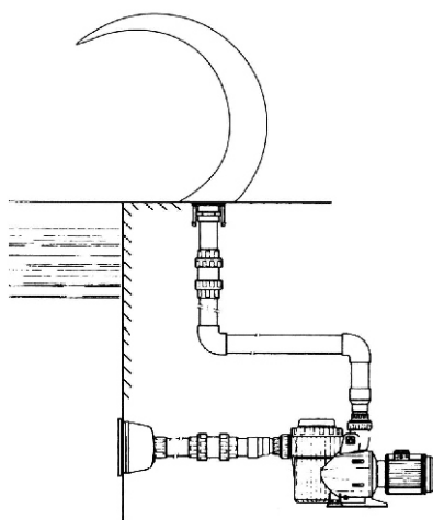
Nákres propojení Connection drawing
